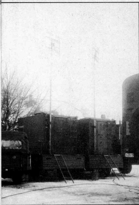
▲ LES ANTENNES POUR LES FAISCEAUX HERTZIENS SONT RAPIDEMENT MONTÉES SUR LES CAMIONS RÉPARTITEURS.
