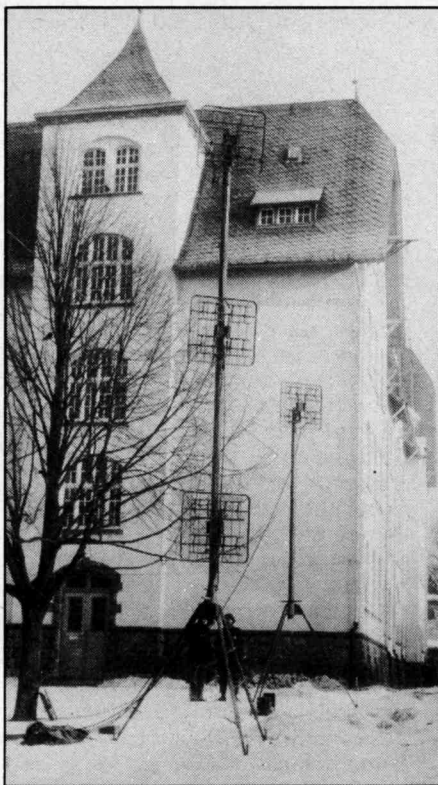
▲ VOICI D'AILLEURS LES ANTENNES DISPOSÉES PAR LE 4 TTR À AROLSSEN.
